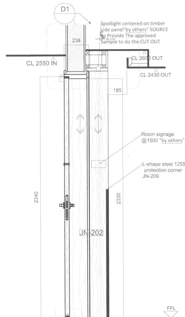
D1 D2 SC1 Section
